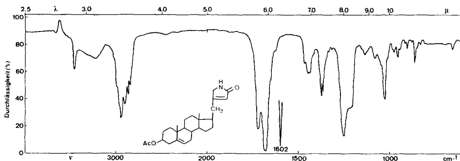
Fig. 1. IR.-Spektrum von 4'-[(3β-Acetoxy-androst-5-en-17β-yl)methyl]-3'-pyrrolin-2'-on ( 14 ) in \text{CHCl}_3
