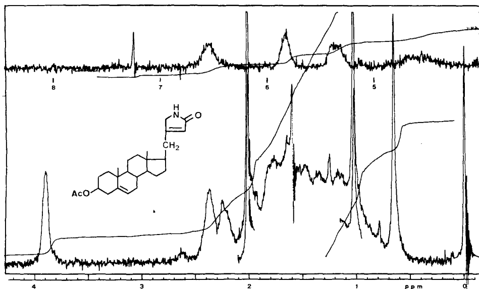
Fig. 2. (60-MHz)-NMR.-Spektrum von 4'-[(3β-Acetoxy-androst-5-en-17β-yl)methyl]-3'-pyrrolin-2'-on ( 14 ) in \text{CDCl}_3
